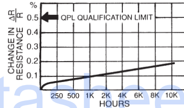
LIFE TEST
