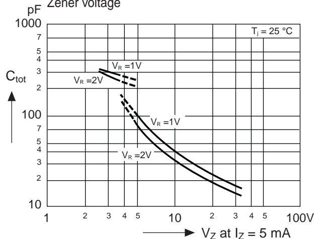
Capacitance versus Zener voltage
